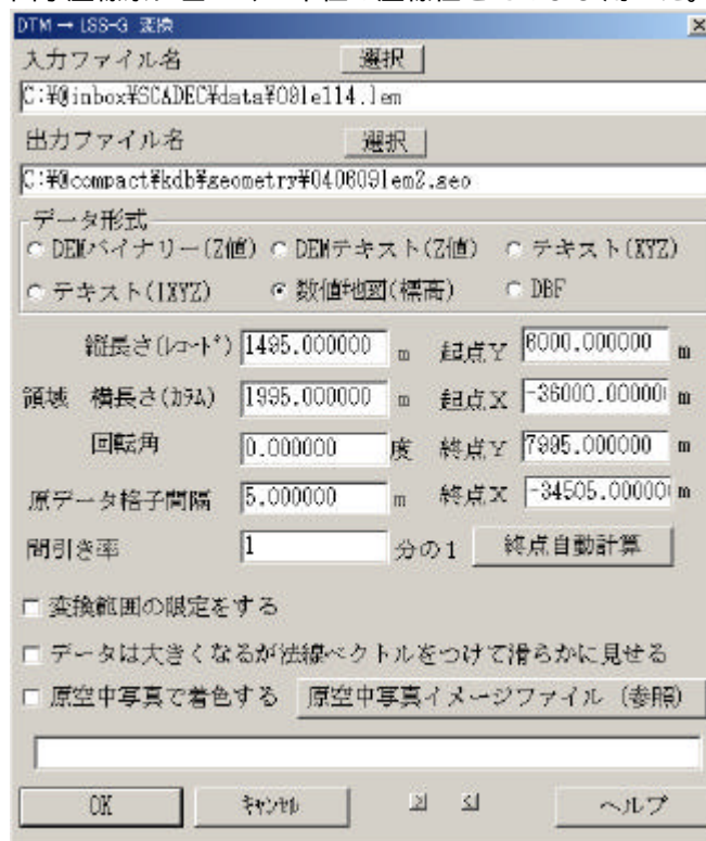
図1 地形のコンバータにおけるパラメータ設定部
