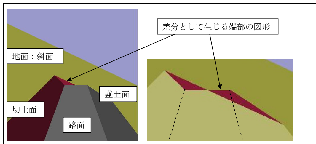
図2-3 地形と構造物の図形演算において端部に自己交差する図形が生じる例 例えば、地形の上に、切土・盛土による法面を有する道路を造成する場合、端部に、差分として振れた図形が生じる場合がある（図2-3）。これを表・裏で複数の面に分割し、表側を地形の上に露出した路面の端面として、また裏側を地形の下に埋没した路面の端面
